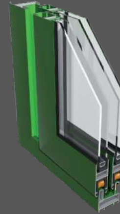
SA 27 & 27 SLIM-INTERLOCK
