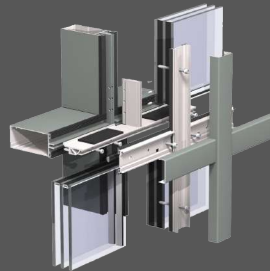
REYNAERS CONCEPTWALL 50
